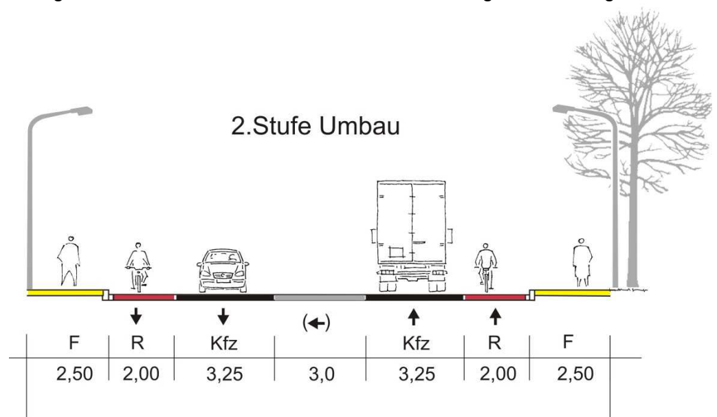
Abb. 62 Gestaltungsvorschlag für die Leerer Landstraße (2. Stufe)
