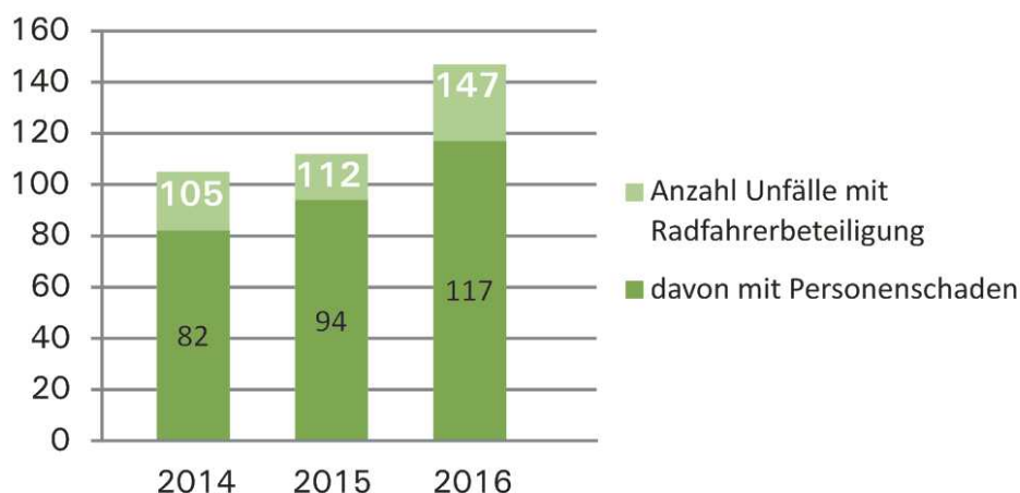
Abb. 18 Unfallentwicklung im Radverkehr in Aurich
