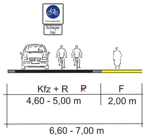
Abb. 58 Umsetzung einer Fahrradstraße Am Neuen Hafen
