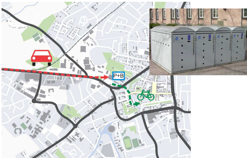
Abb. 76 Mögliche P + B Anlage an der Sparkassen-Arena
