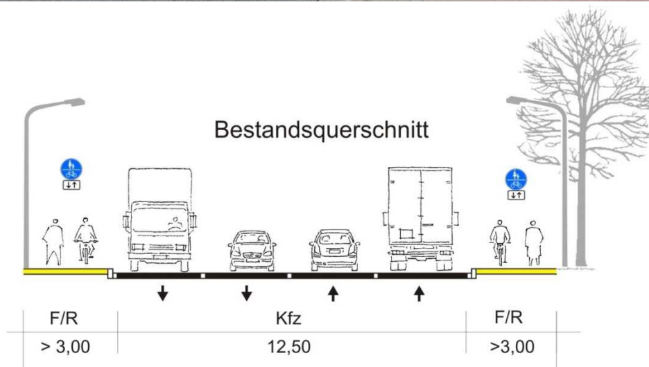
Abb. 60 Querschnitt im Bestand in der Leerer Landstraße
